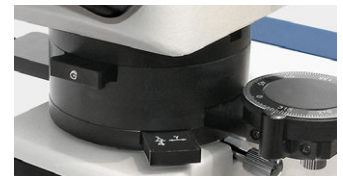
Lente de Bertrand, deslizamiento \lambda , analizador giratoria (360°) (extraíble)
